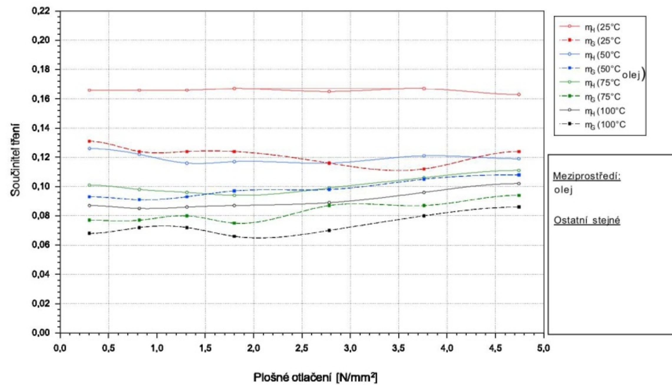
Obr. 72 Hodnota tření ZX-530 při mazání olejem; měřená po záběhu
