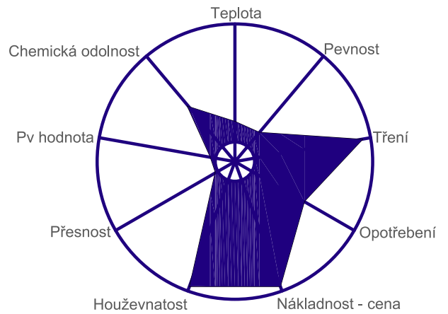
Přehled vlastností materiálu PTFE
