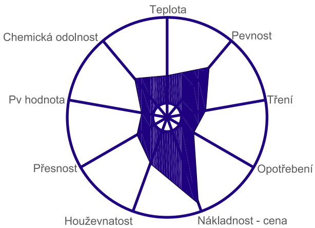
Přehled vlastností materiálu Bronz
